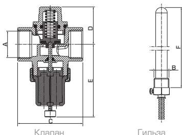
Клапан
