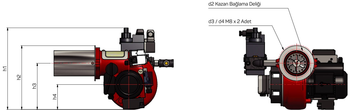
Kazana Bağlama Ölçüleri Connection Sizes to the Boiler Размеры Связывания Котла
